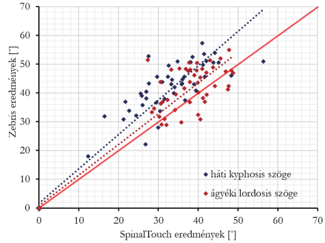
4. ábra. Mérérendszerek összehasonlítása lineáris regresszió alkalmazása esetén
